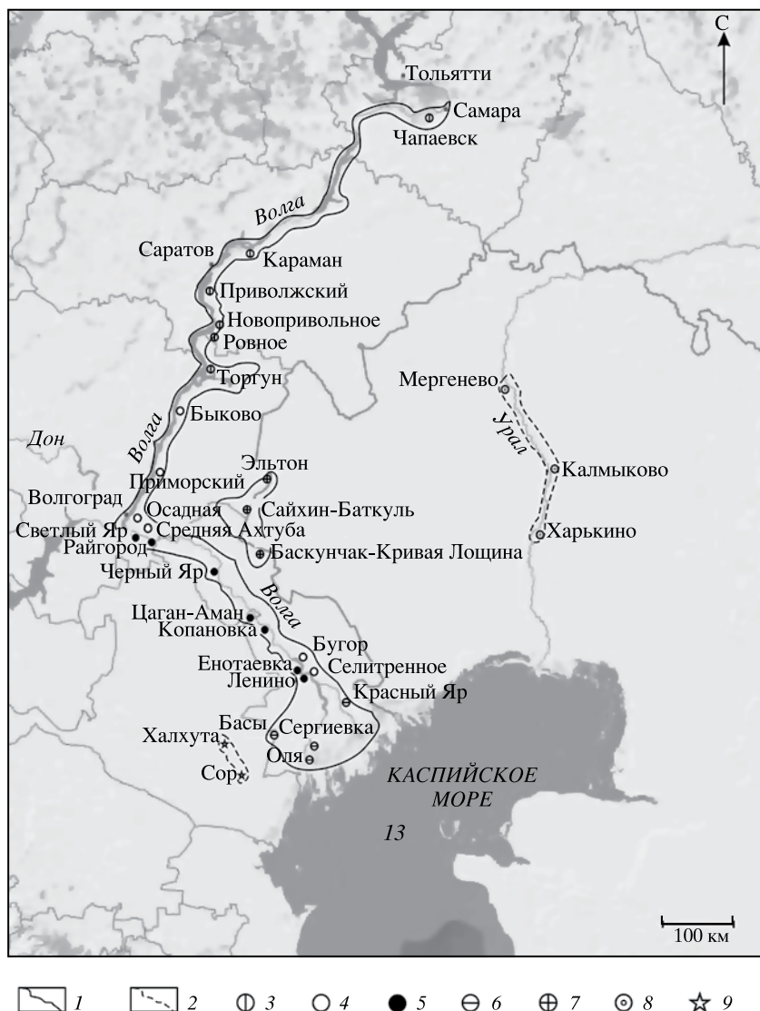
Рис. 1. Схема расположения разрезов шоколадных глин Предполагаемое распространение глин: 1 – сплошное, 2 – прерывистое; местоположение опорных разрезов: 3 – Среднее Поволжье, 4 – левобережье р. Волги, 5 – Правобережье р. Волги, 6 – дельта р. Волги, 7 – депрессии Кайсацкое – Эльтон – Верхний Баскунчак, 8 – долина р. Урал, 9 – Калмыкия
