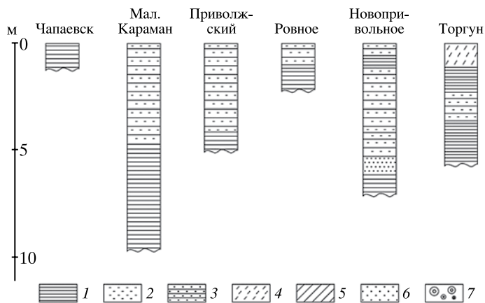
Рис. 2. Разрезы Среднего Поволжья Глины: 1 – шоколадные, 2 – с алевритом, 3 – с песком; 4 – супесь; 5 – суглинок; 6 – песок и галька; 7 – раковины моллюсков
