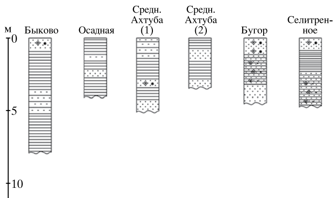
Рис. 3. Разрезы правобережья р. Волги Здесь и далее усл. обозначения см. рис. 2
