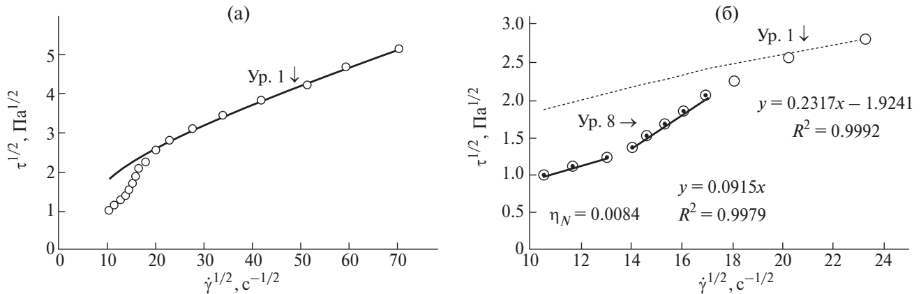
Рис. 4. Зависимость напряжения сдвига от скорости сдвига в корневых координатах для мицеллярного раствора СТАВ/NaSal с концентрацией сурфактанта CD(M) = 0.08 . а – на полном интервале скоростей сдвига; б – на интервале низких скоростей сдвига.
