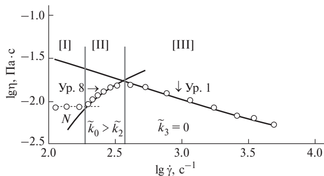
Рис. 3. Зависимость вязкости от скорости сдвига в двойных логарифмических координатах для мицеллярного раствора СТАВ/NaSal с концентрацией сурфактанта C_D (M) = 0.08 . Экспериментальные данные из работы [20].
