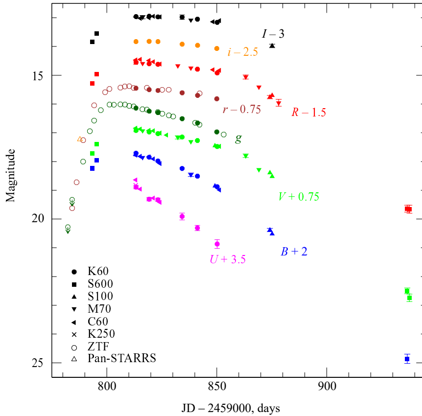
Рис. 2. Кривые блеска SN 2022prv в полосах U , B , V , R , I , g , r , i . Названия фильтров и смещения соответствующих кривых приведены на графике. Форма символов показывает источники данных, их обозначения соответствуют приведенным в тексте. Верхние пределы блеска показаны стрелками вниз.
