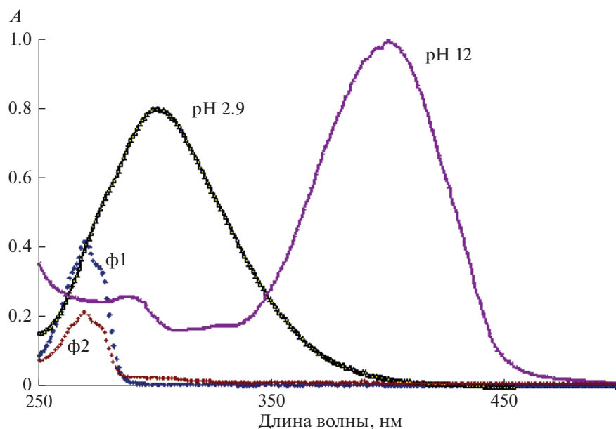
Рис. 1. Оптическая плотность A (отн. ед.) исходного раствора фенола 0.265 ммоль/л ( \phi 1 ); того же раствора, смешанного с азотной кислотой pH 2.7 в соотношении 1 : 1 ( \phi 2 ); раствора фенола 0.265 ммоль/л, смешанного с АПВ, обработанной излучением генератора ИР10 в течение 15 мин 1 : 1 на второй день после смешивания (pH 2.9); раствора (pH 2.9), в который на второй день после смешивания добавлены кристаллы щелочи NaOH (pH 12).
