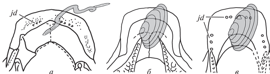
Рис. 7. Возможные способы захвата пищевых объектов различным диптеридными двоякодышащими: а — захват удлиненного объекта с помощью короткого симфиза у Anchidipterus ; б, в — захват изометричного объекта с помощью значительной поверхности контакта удлиненного симфиза: б — Dipterus (из: Jarvik, 1967), в — Orlovichthys (из: Крупина, 1980). Эффективность захвата увеличивали челюстные зубчики на оральной поверхности нижней челюсти. Обозначение: jd — челюстные зубчики.
