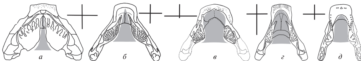
Рис. 6. Реконструкция площади “поршня гиоидного насоса” (обозначена серой заливкой) и конфигурация симфизной пластины нижних челюстей у различных девонских двоякодышащих (стеносимфизный и платисимфизный типы); крестовидные диаграммы показывают соотношение ширины рта и длины симфизной пластины: a , б , з – стеносимфизный тип, в , д – платисимфизный тип: a – Chirodipterus australis Miles, 1977; б – Dipterus valenciennesi Sedgwick et Murchison, 1828; в – Anchidipterus dariae Krupina, gen. et sp. nov.; з – Rhinodipterus ulrichi Örvig, 1961; д – Orlovichthys limnatis Krupina, 1980 [ a – из Майлса (Miles, 1977); б , з – из Ярвика (Jarvik, 1967); д – из Крупиной (1980)].
