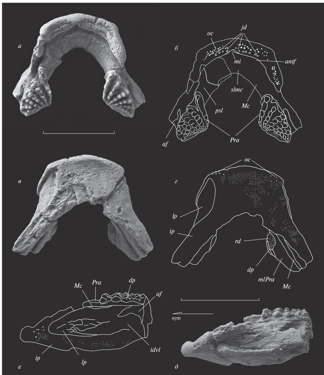
Рис. 2. Anchidipterus dariae Krupina, gen. et sp. nov., голотип КМА/4213, неполная нижняя челюсть: a, б — дорсально, в, г — вентрально, д, е — латерально слева. Стрелка на ( д ) направлена рострально. Обозначения: af — аддукторная яма; antf — передняя борозда, ограничивающая задний край dentale; dp — зубная пластинка; idvl — вертикальная инфраден- тальная пластина; ip — горизонтальная инфраден- тальная пластина; jd — зубчики на dentale; lp — лабиальная ямка; Mc — меккелев хрящ; mi — медиальная вырезка на dentale; mlPra — мезиальные пластины praearticulare; oc — отверстия выхо- да наружных ветвей оральной ветви сенсорного канала; Pra — praearticulare с преартикулярными зубными пластинка- ми; psl — передние (симфизные) пластины praearticulare; rd — участок зубной пластинки, сформированный репаратив- ным дентином; slmc — симфизная пластина меккелева хряща. Масштабная линейка 10 мм.
