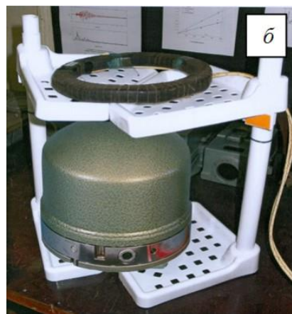
Рисунок 1. Общий вид лабораторного оборудования эксперимента по проверке воздействия магнитного поля на сейсмометры: (а) – СМ-3КВ; (б) – STS-2
