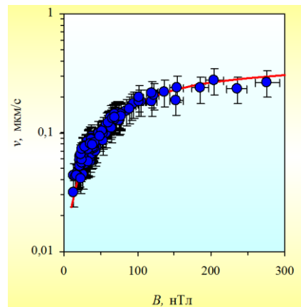
Рисунок 3. Зависимость между среднеквадратичной амплитудой вариаций микросейсмического фона \nu , наведенных в период геомагнитных возмущений, и амплитудой геомагнитного импульса B
