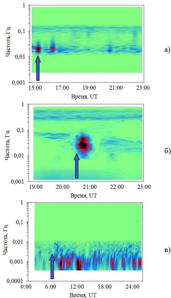
Рисунок 2. Примеры вариаций сейсмического фона ( \nu ) в период геомагнитных возмущений (начало обозначено вертикальными залитыми стрелками). Параметры геомагнитных возмущений: (а) – 30.04.2008 г. – K=4 ; B=37 нТл; (б) – 26.12.2015 г. – K=5 ; B=67 нТл; (в) – 29.09.2011 г. – K=6 ; B=120 нТл.
