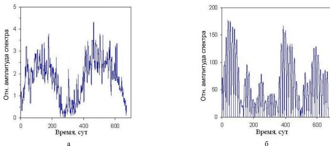
Рисунок 7. Модуль спектральных составляющих геомагнитных вариаций с периодами: а – 1 сутки; б – 27 суток
