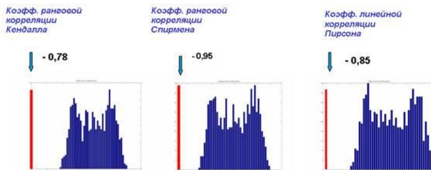
Рисунок 13. Результаты оценки тесноты корреляционной зависимости и неслучайности между магнитным типпером и уровнем подземных вод
