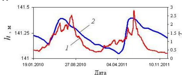
Рисунок 12. Сопоставление вариаций магнитного типпера (1) и уровня подземных вод (2) на ГФО МНВ
