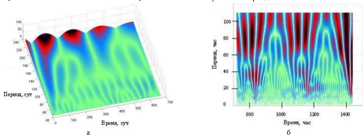
Рисунок 6. Скалограммы геомагнитных вариаций за 2011 – 2012 гг. в интервале периодов: (а) 60 – 240 сут. (за февраль 2011 г.); (б) 0,5 – 110 сут.
