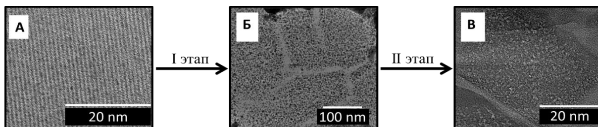
Рисунок 1. Микроснимки образцов, полученных в ходе различных этапов обработки: исходный цеолит CBV100 (А); образец после кислотной обработки с дефектами цеолитной структуры (Б); образец после нескольких часов гидротермальной обработки (В).
